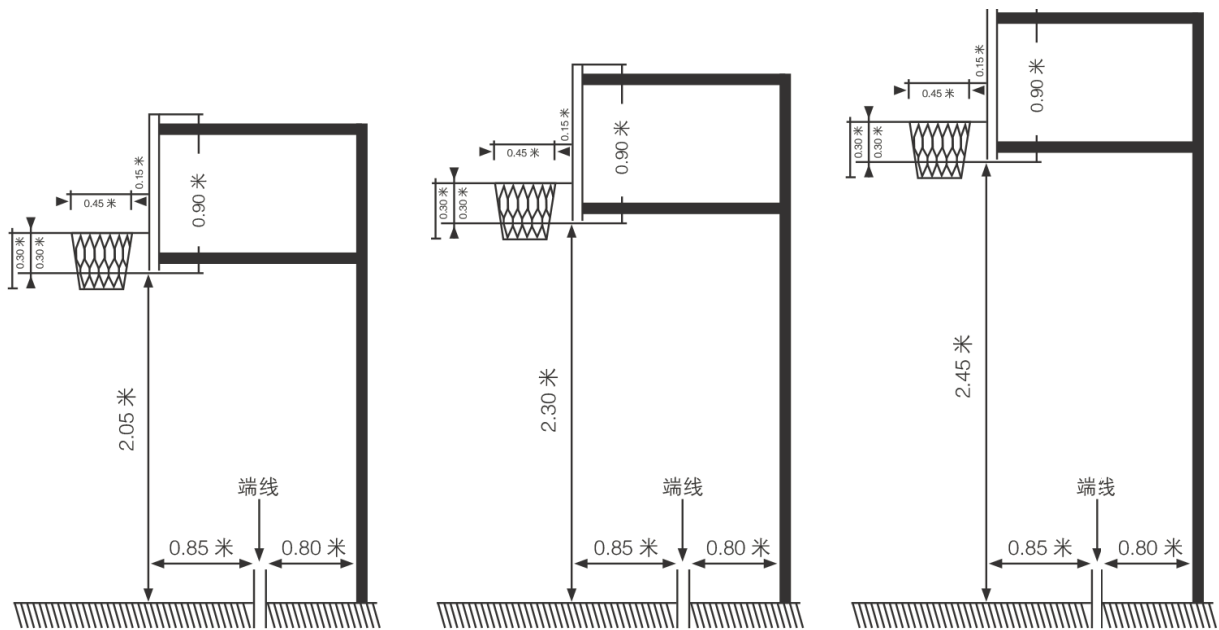
图3 小篮球篮架球篮尺寸图
