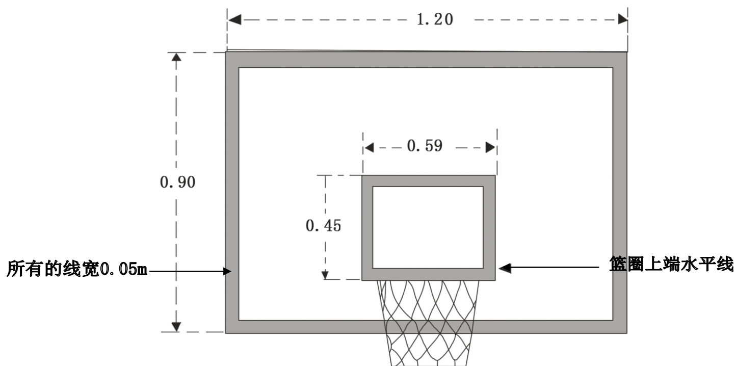
图 2 小篮球篮板尺寸图
