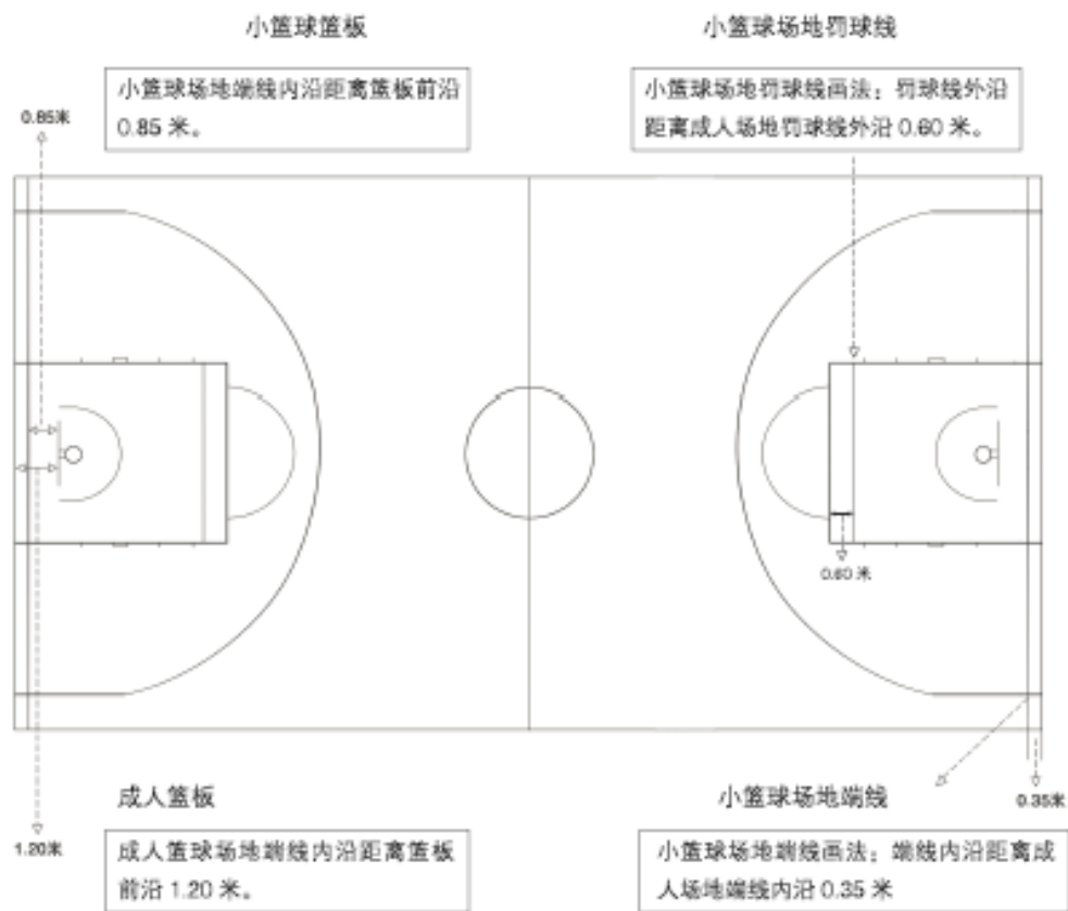
图 35 成人篮球比赛场地套画小篮球场地尺寸图
