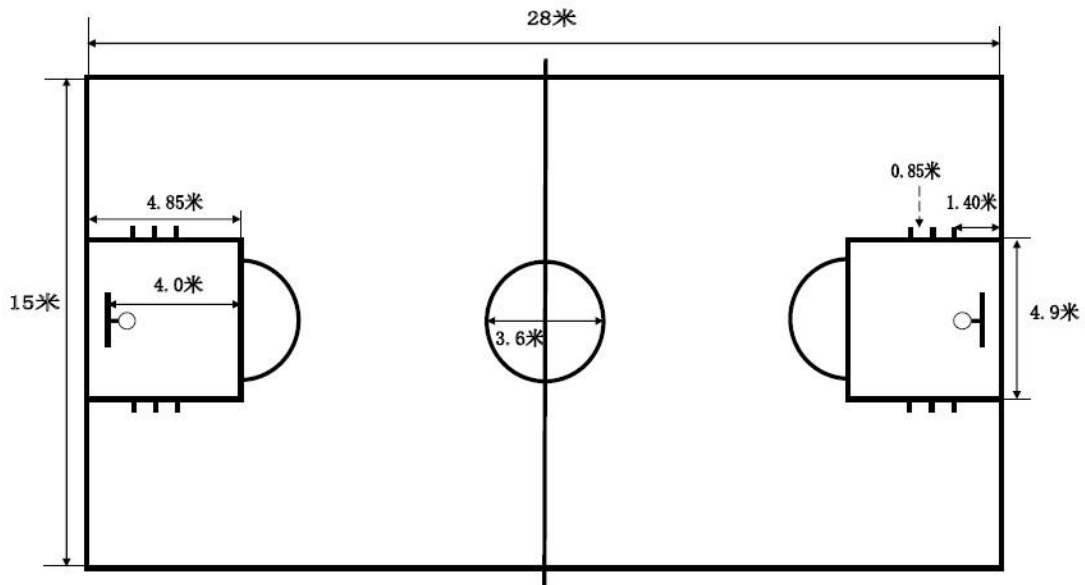
图 1 小篮球场尺寸图
